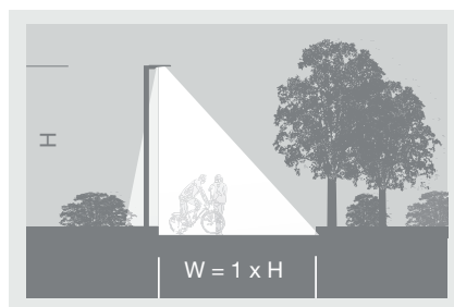
P1.0a – Für schmale Straßen und Wege: Asymmetrisch, extrem breit strahlend
